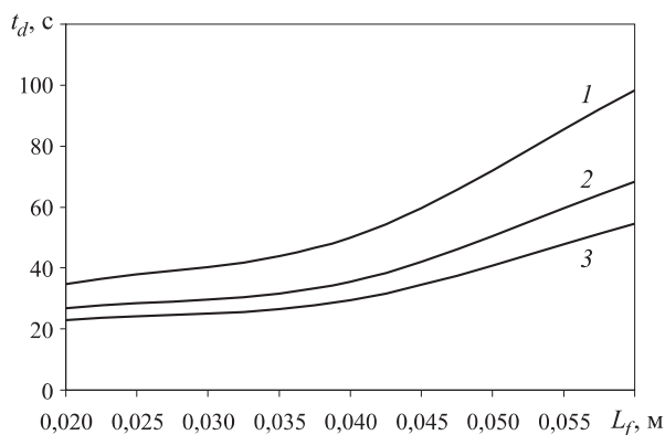
Рис. 6. Зависимость времени подавления реакции термического разложения от толщины ЛГМ [94] при L_w = 0,002 \text{ м} : 1 — листья березы; 2 — хвоя сосны; 3 — хвоя ели
