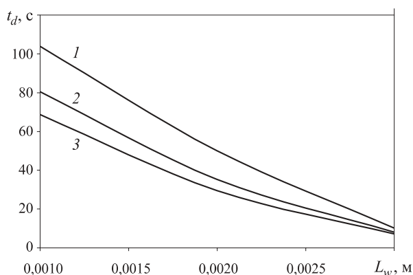
Рис. 7. Зависимость времени подавления реакции термического разложения от толщины слоя ЛГМ-вода при L_f = 0,04 \text{ м} [94]: 1 — листья березы; 2 — хвоя сосны; 3 — хвоя ели
