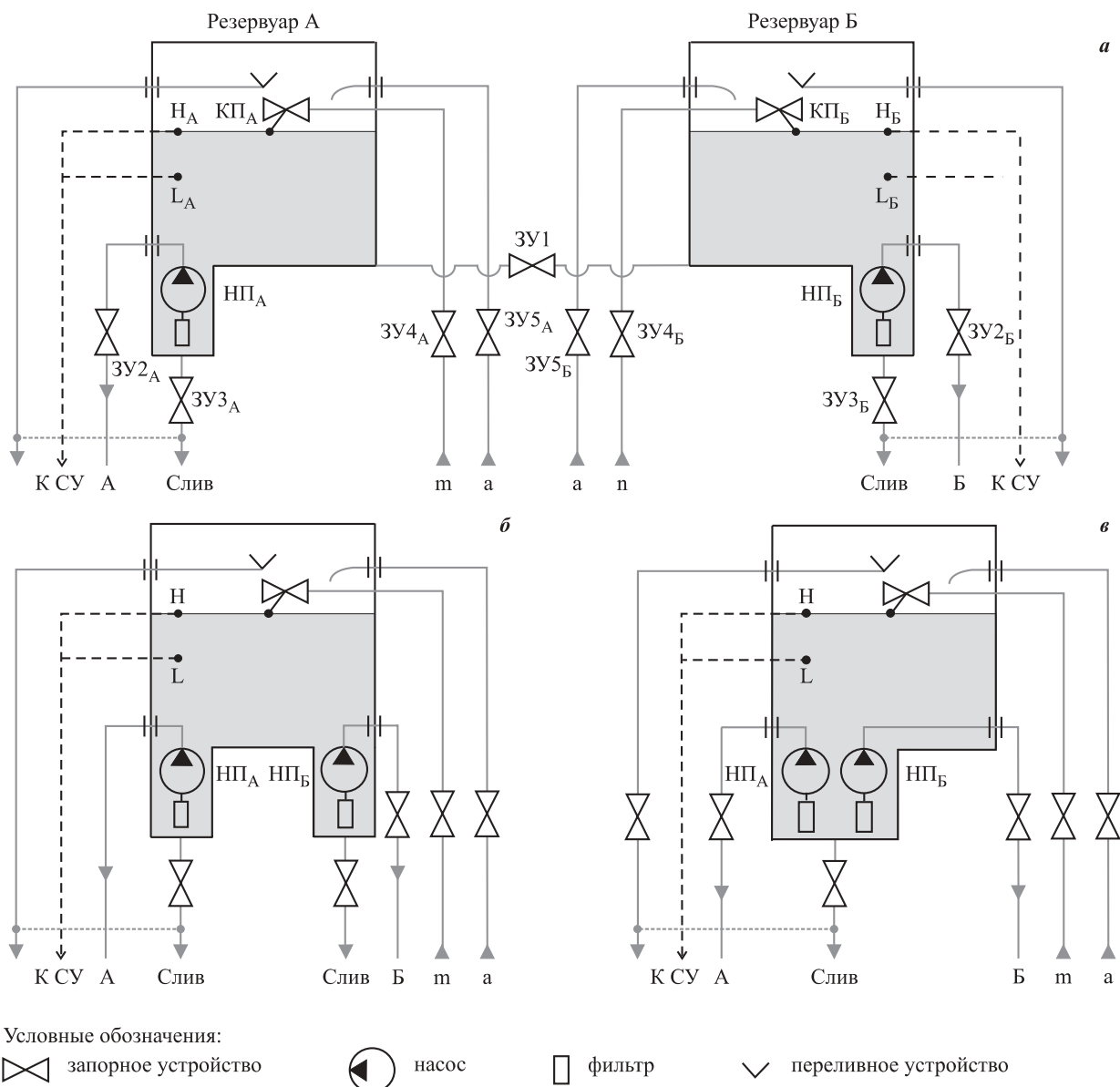
Рис. 4. Схема противопожарного водоснабжения: а — ВПВ из двух пожарных резервуаров или ВПВ, совмещенный с АУП, и/или с ХПВ, и/или с НПВ, или с технологическим водопроводом; б — ВПВ или ВПВ, совмещенный с АУП, и/или с ХПВ, или с технологическим водопроводом из одного пожарного резервуара (при наличии приемка для каждого пожарного насоса); в — то же, при наличии общего приемка для всех пожарных насосов
