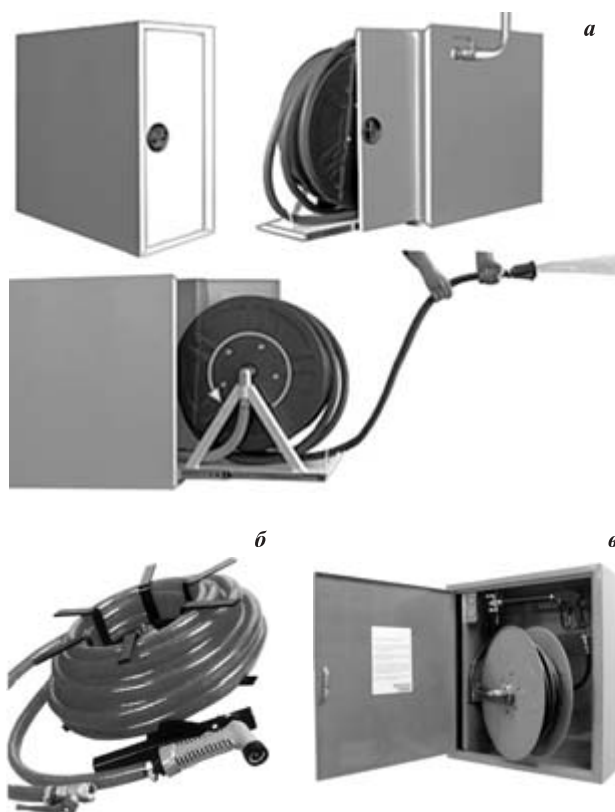
Рис. 2. Внешний вид барабанного ПК-м [22] (а), ПК-м-ТРВ [23] (б) и ПК-м-ТРВ высокого давления [24] (в)
