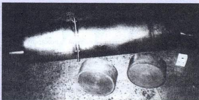
Рис. 1. Модифицированный глушитель с каталитическими блоками КНГ-220/2-186
