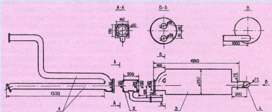
Рис. 2. Схема газовыпускного тракта двигателя пожарного автомобиля АЦ-40 (43202) 186: 1 — сочлененные выпускные трубы; 2 — устройство всасывающее газоструйное (УВГ-1); 3 — серийный глушитель шума автомобиля Урал-4320, вместо которого монтируется КНГ-220/2-186; 4 — выпускная труба.
