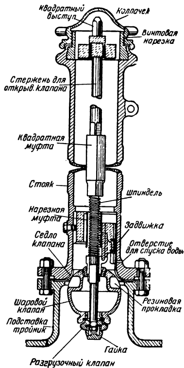
Рис. 14. Подземный гидрант московского типа.
