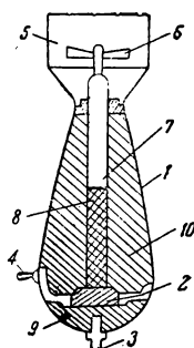
Рис. 40. Термитная бомба сосредоточенного действия:
