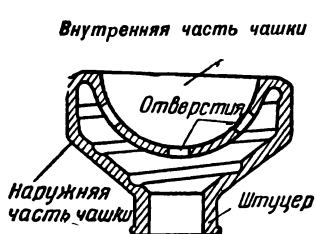
Рис. 34. Водораспылитель системы П. И. Снегирева.
