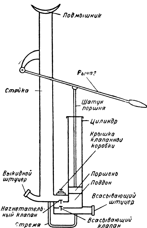
Рис. 20. Гидропульт-костыль.
