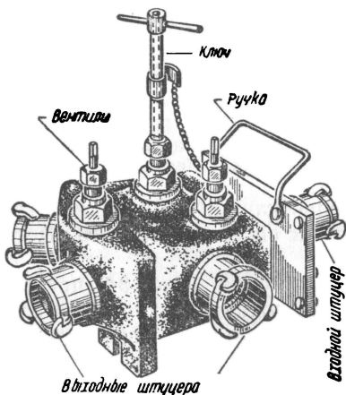
Рис. 37. Трехходовой кран.
