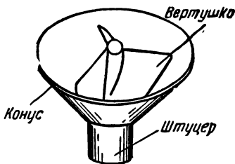
Рис. 35. Водораспылитель системы Пегова.
