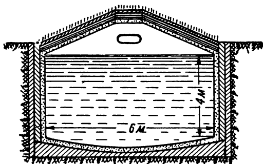
Рис. 17. Подземное водохранилище.
