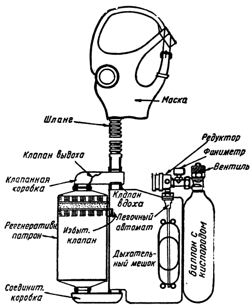
Рис. 33. Кислородный (изолирующий) прибор КИП-3.
