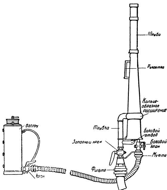
Рис. 18. Воздушно-пенный ствол «Комета».
