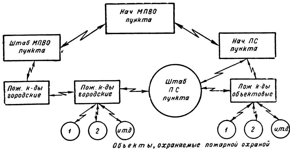
Рис. 11. Схема пожарной связи на пункте МПВО.
