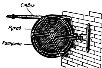
Рис. 16. Рукавная катушка для внутреннего пожарного крана.
