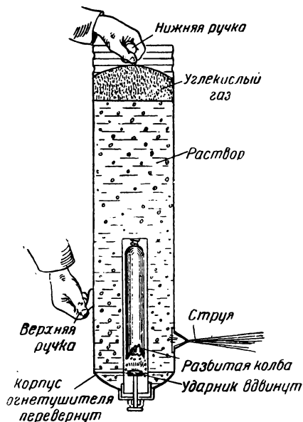
Рис. 25. Действие пенного огнетушителя «Богатырь» № 1.
