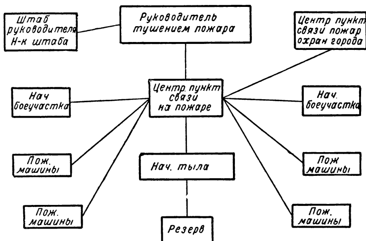
Рис. 49. Схема организации связи на пожаре (средства: телефон, звуковая и световая сигнализация, посыльные и радио).
