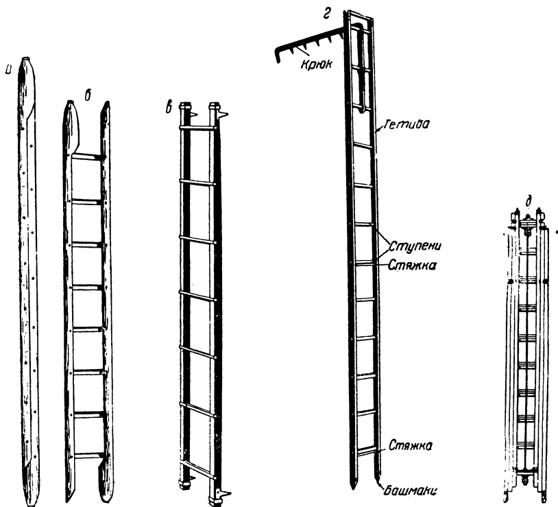
Рис. 31. Пожарные лестницы:
