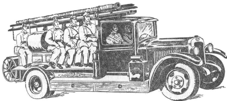
Рис. 30. Автонасос ЗИС-11.
