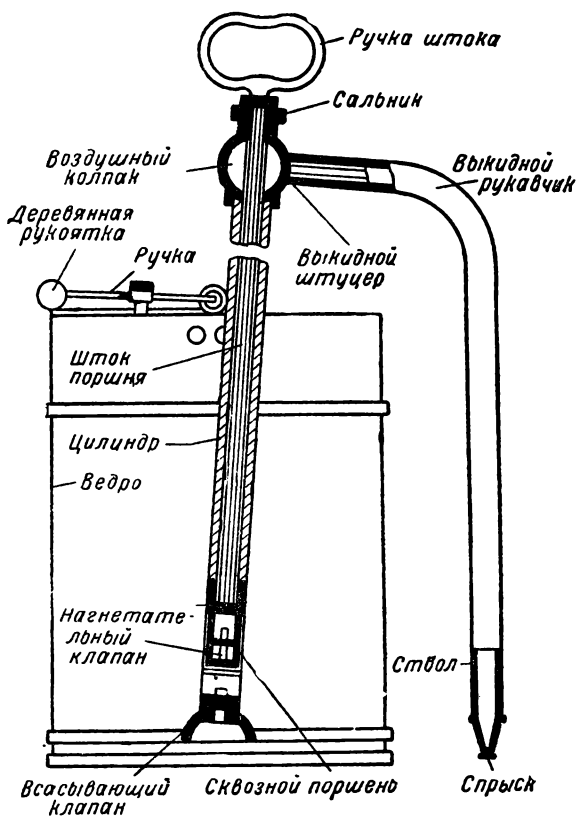
Рис. 19. Гидропульт-ведро.
