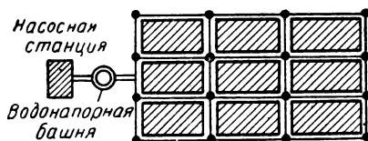
Рис. 12. Схема кольцевой сети водопровода.
