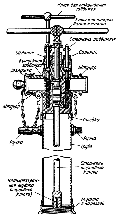
Рис. 15. Стендер московского типа.
