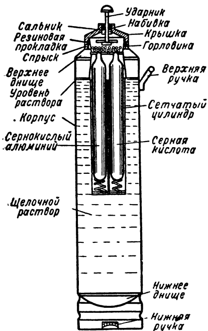
Рис. 24. Густопенный огнетушитель «Богатырь» № 3.
