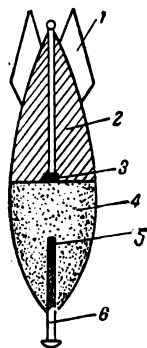
Рис. 41. Электронно-термитная бомба сосредоточенного действия:
