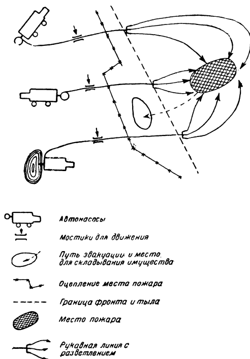
Рис. 50. Схема развертывания на пожаре.
