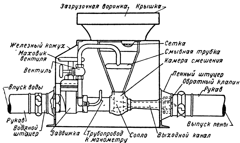
Рис. 28. Пеногенератор ВАТО.
