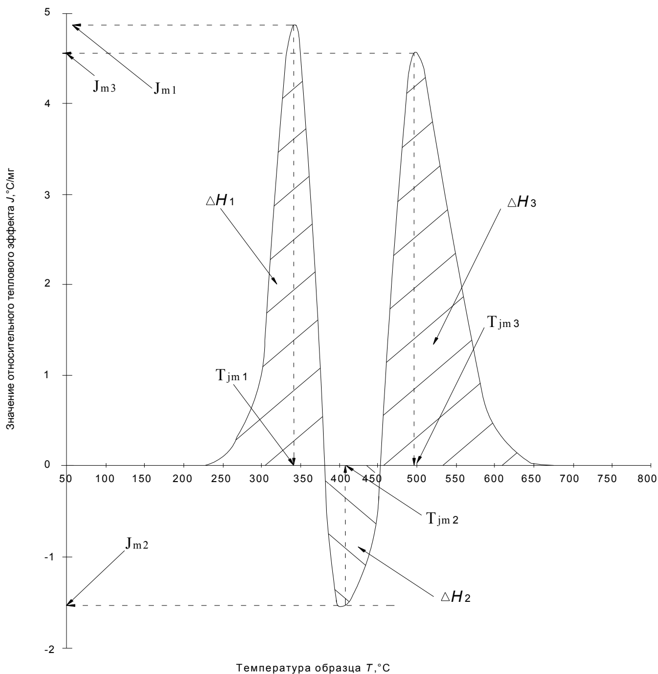
Рисунок А.3 – Пример определения значений относительного теплового эффекта по ДТА – зависимости
