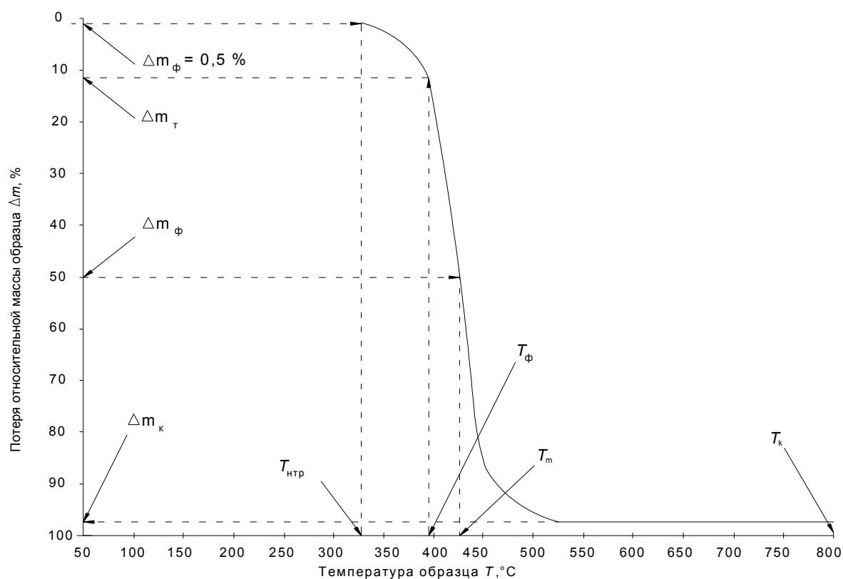
Рисунок А.1 – Пример определения значений потери относительной массы образца по ТГ - зависимости
