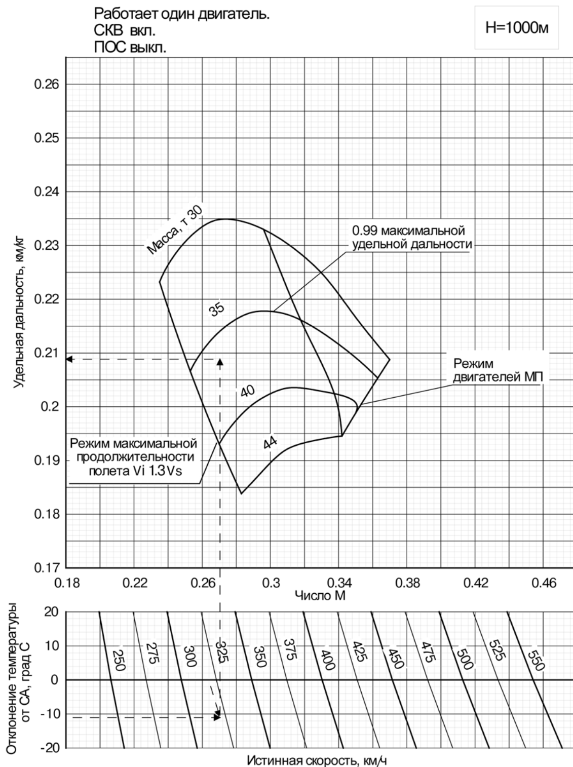
Рис. 38 Удельная дальность
