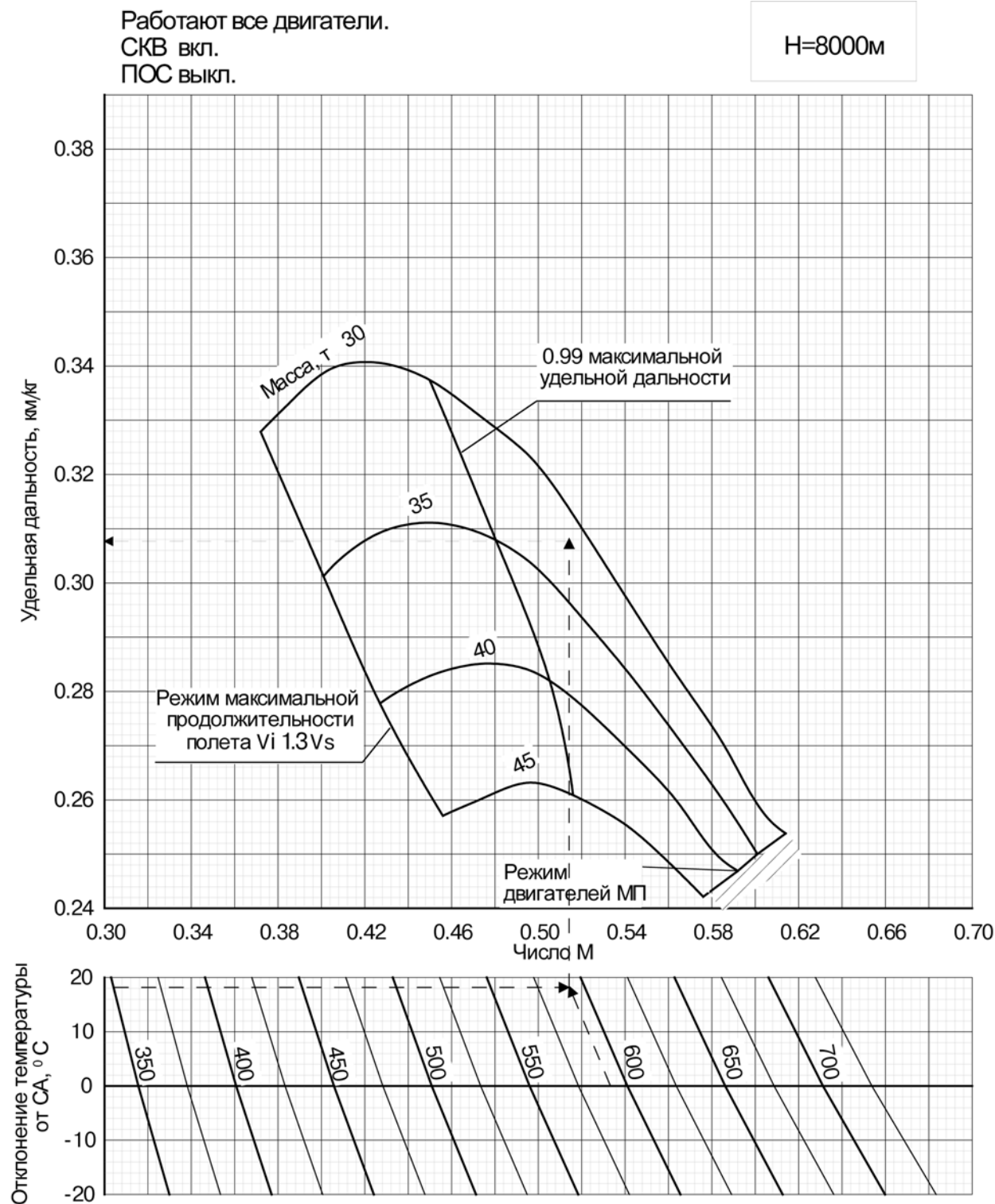
Рис. 36 Удельная дальность
