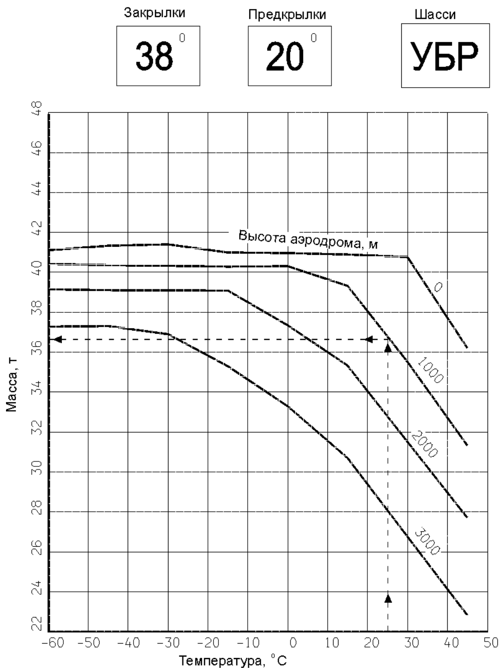
Рис. 10 Максимальная взлетная масса, ограниченная градиентом набора высоты при взлете с воды
