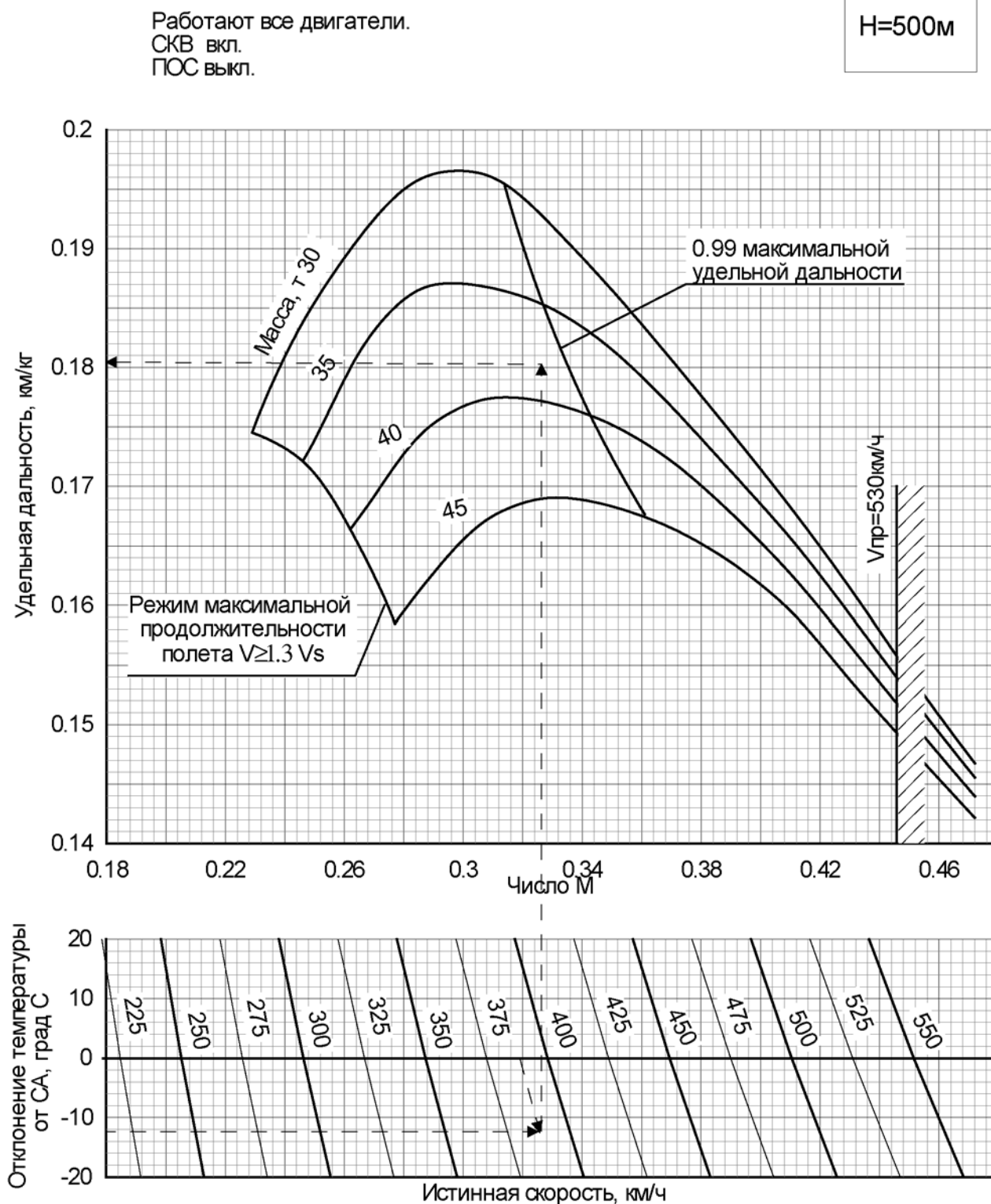
Рис. 28 Удельная дальность
