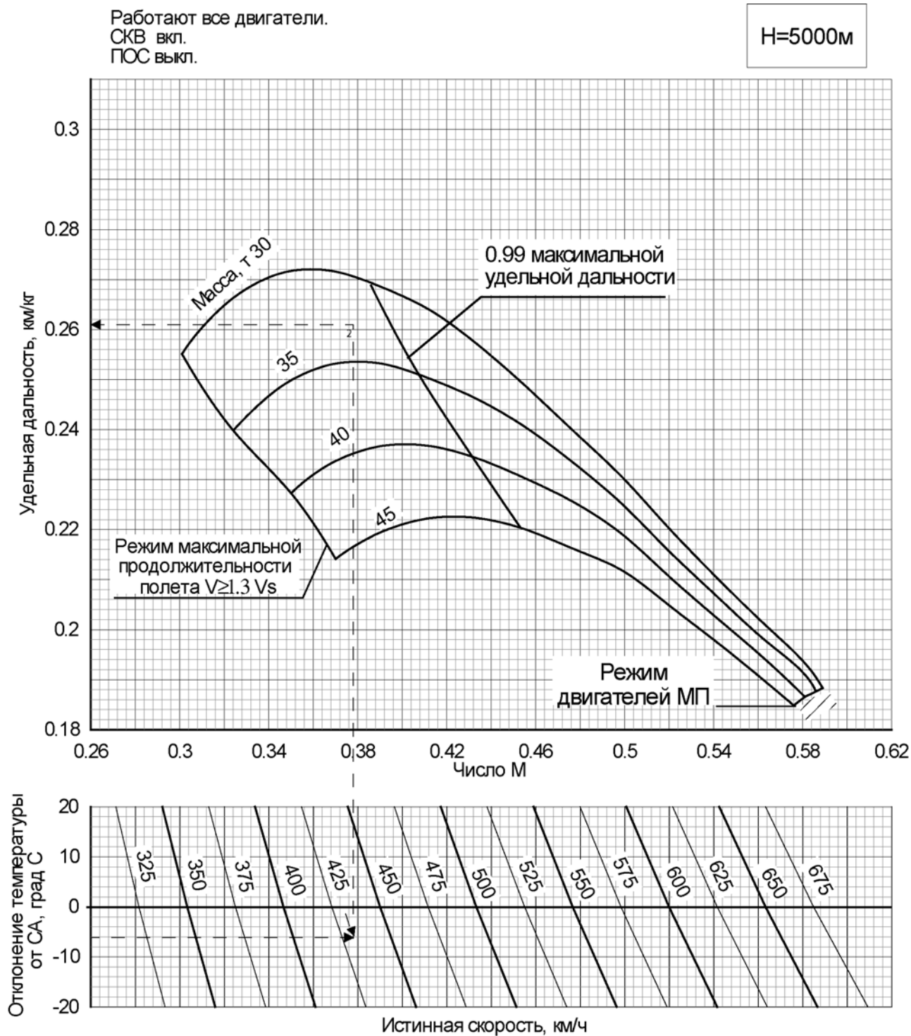
Рис. 33 Удельная дальность
