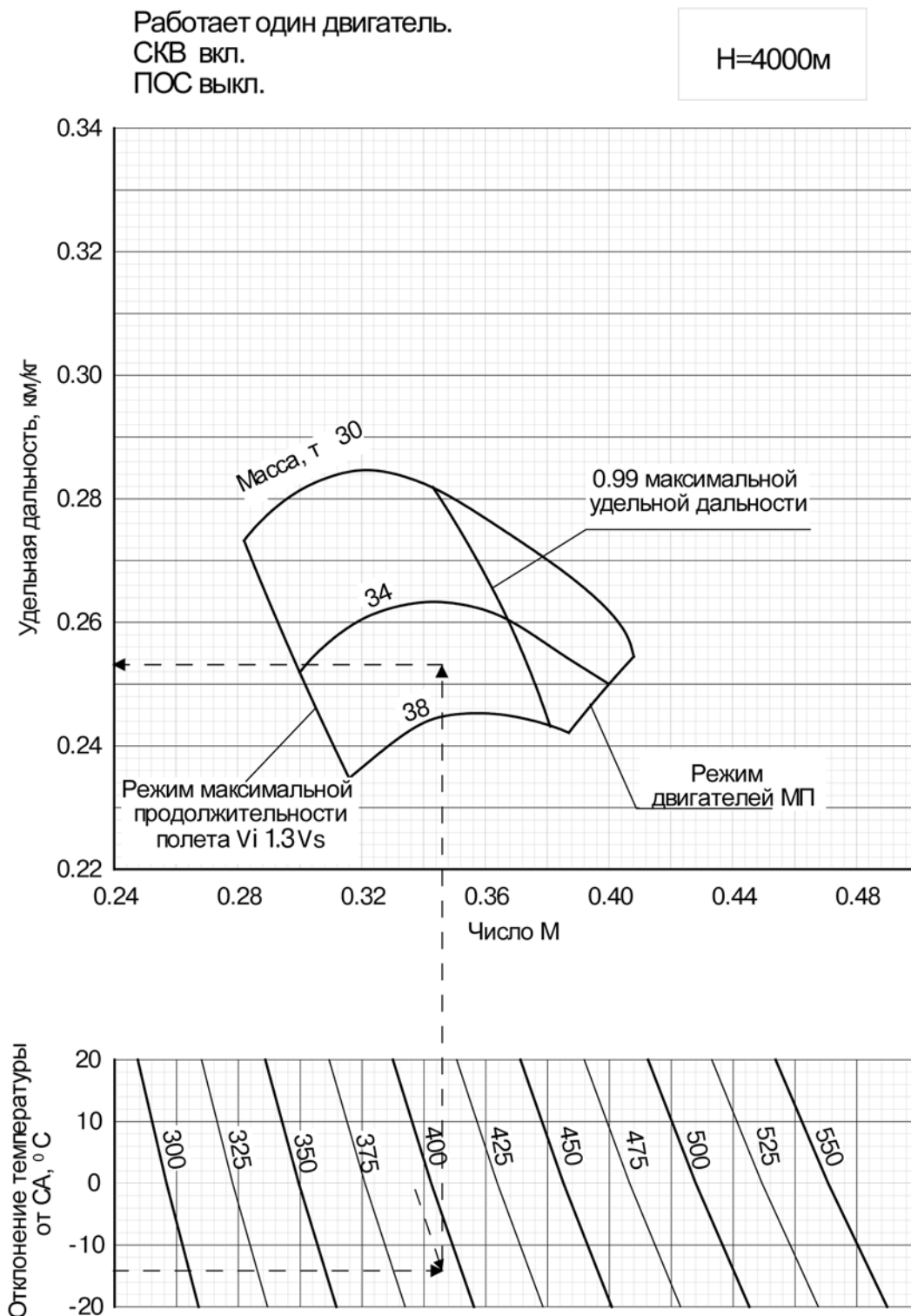
Рис. 41 Удельная дальность
