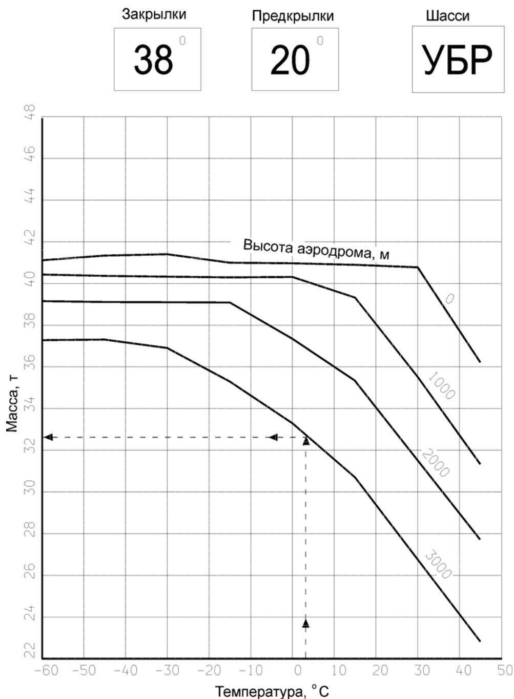
Рис. 52 Максимальная посадочная масса, ограниченная градиентом набора высоты при уходе на второй круг
