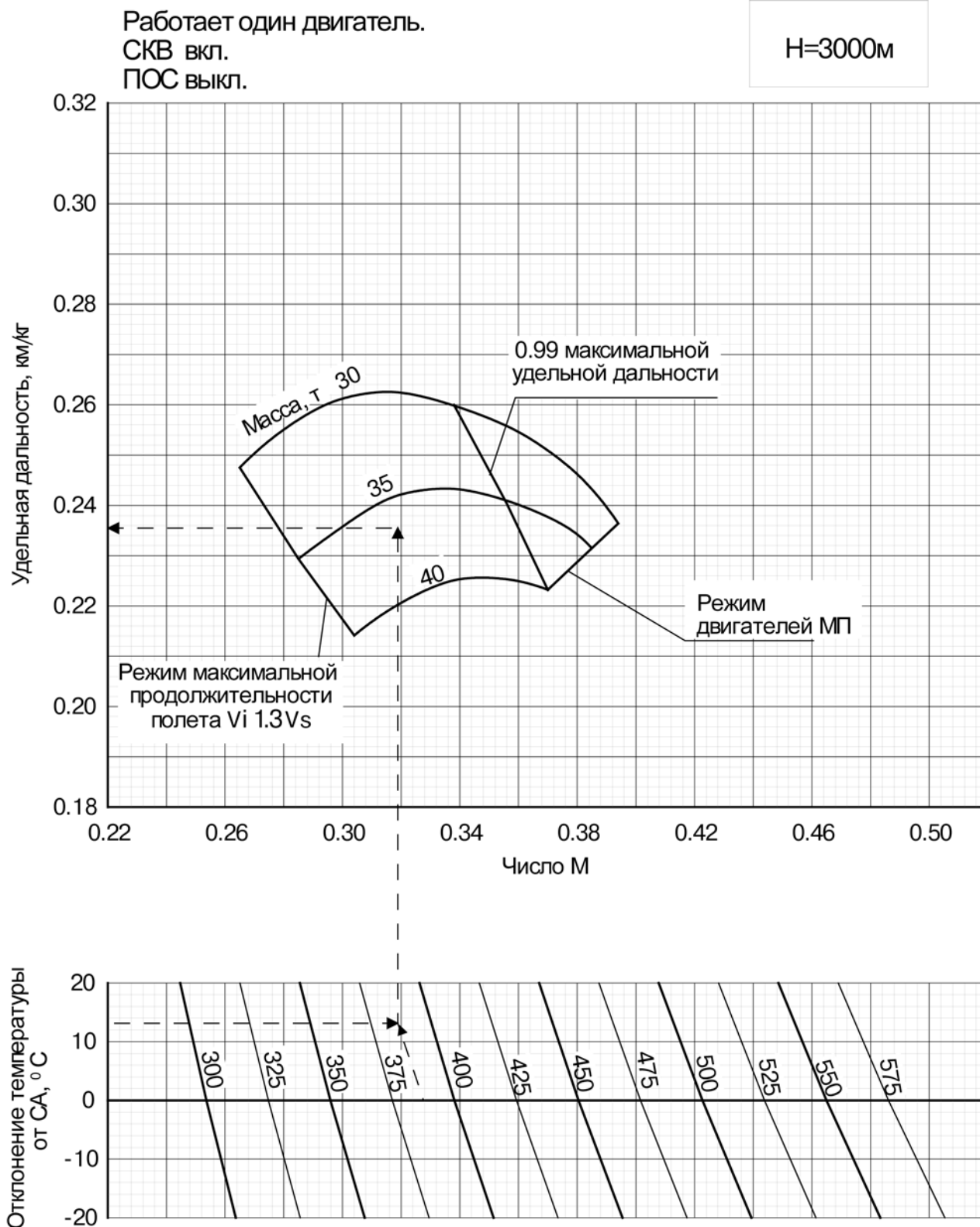
Рис. 40 Удельная дальность
