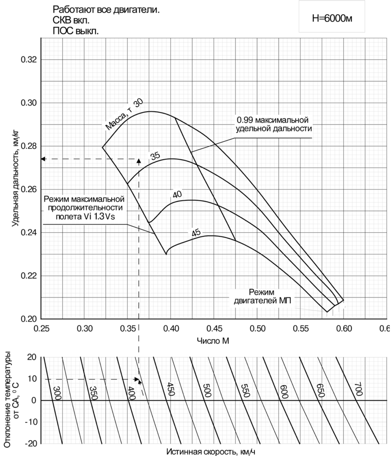
Рис. 34 Удельная дальность
