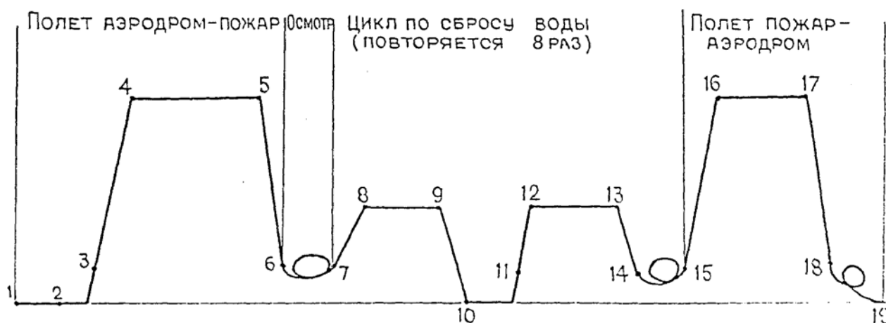
Рис. 2 Профиль полета
