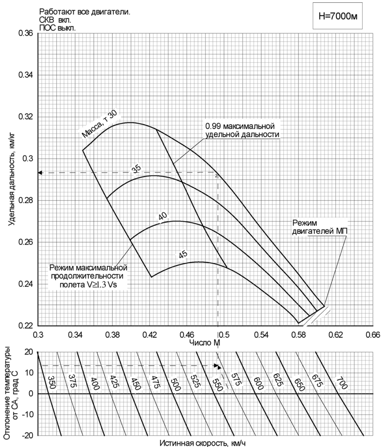
Рис. 35 Удельная дальность
