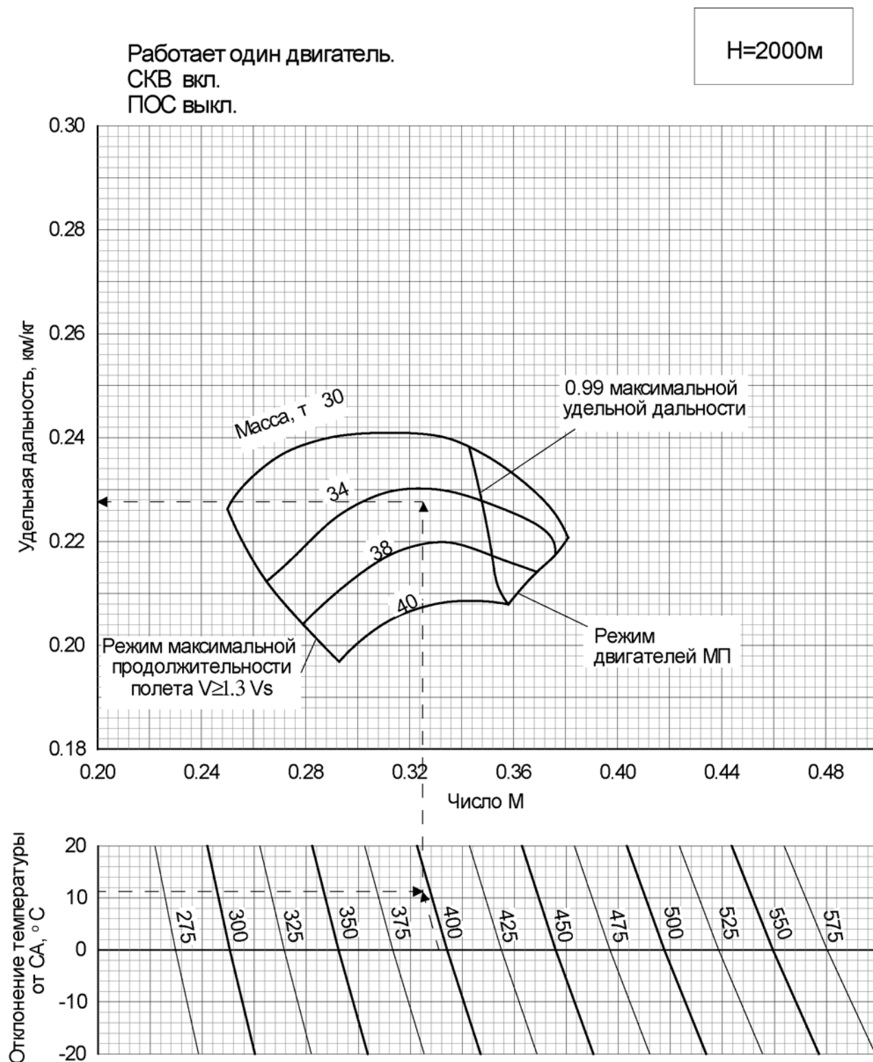
Рис. 39 Удельная дальность
