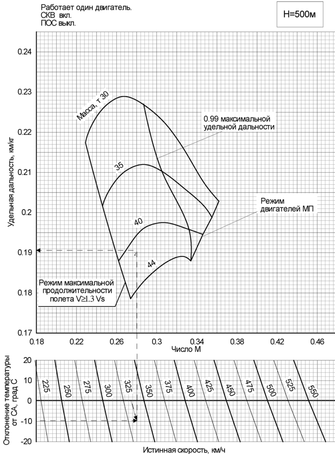
Рис. 37 Удельная дальность
