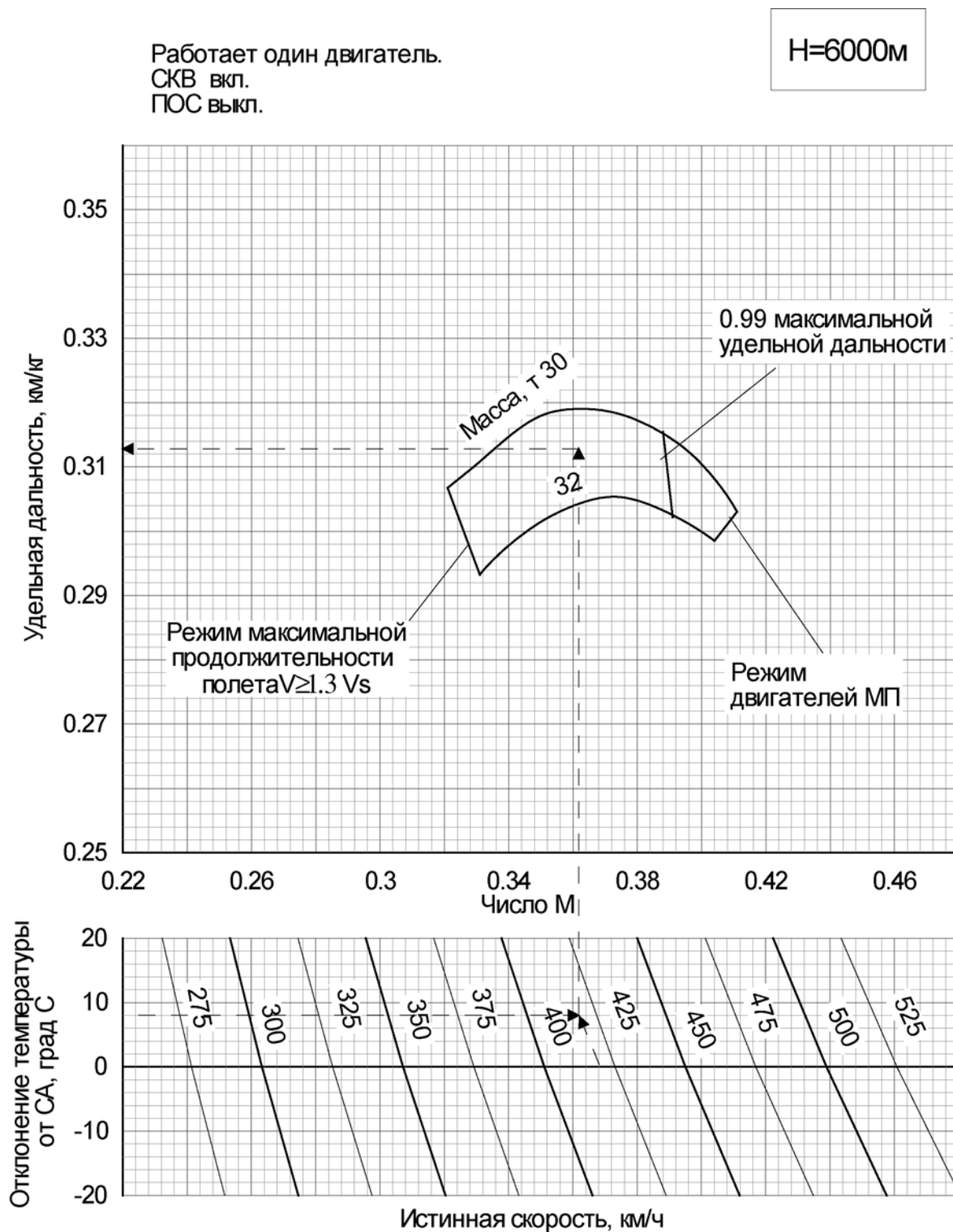
Рис. 43 Удельная дальность
