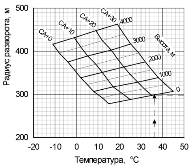
Рис. 56 Радиус разворота при тушении пожара
