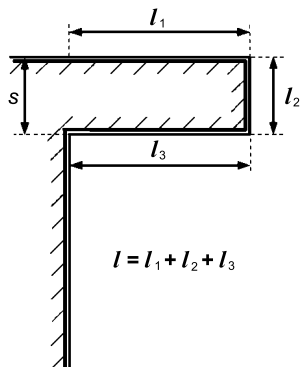
Рисунок 7.15 – Петля в токоотводе
