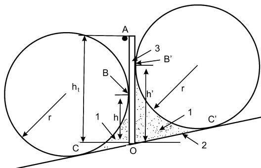
1 – зона защиты; 2 – уровень отсчета; 3 – строжневой молниеприемник; r – радиус катящегося шара; h_t , h' – высоты молниеприемников; h – высота молниеприемного стержня (мачты, троса) над расчетным уровнем; A – трос; B , C , B' , C' – точки касания катящегося шара ( h < h_t , h' < h_t )
