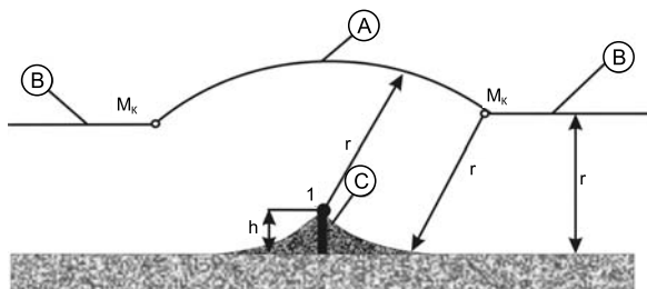
1 – тросовый молниеприемник
