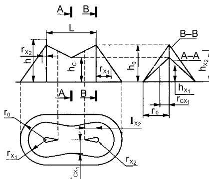
Рисунок 10.4 – Зона защиты двойного стержневого молниеотвода
