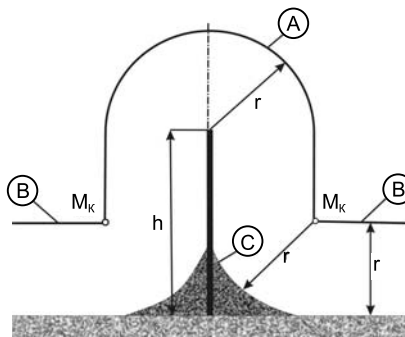
Рисунок 7.7 – Зона защиты башенного молниеотвода ( h > r )
