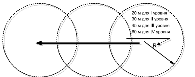
Рисунок 7.10 – Качение сферы радиусом уровня молниезащиты на ровной поверхности
