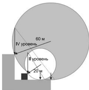
Наиболее опасный объект имеет более сложную молниезащиту
