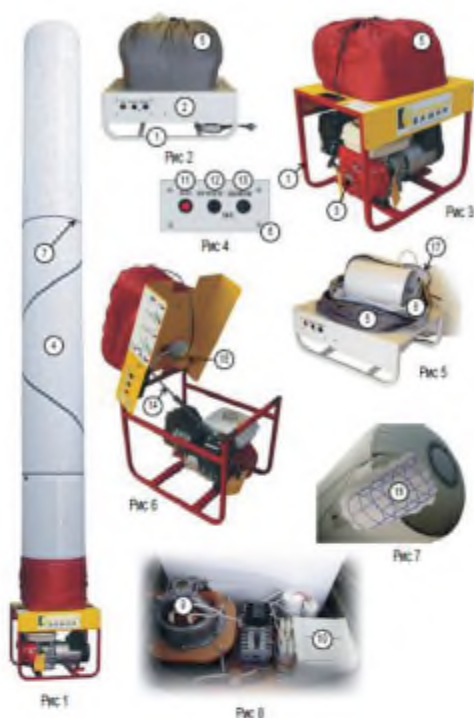
Аварийная мобильная осветительная надувная установка
