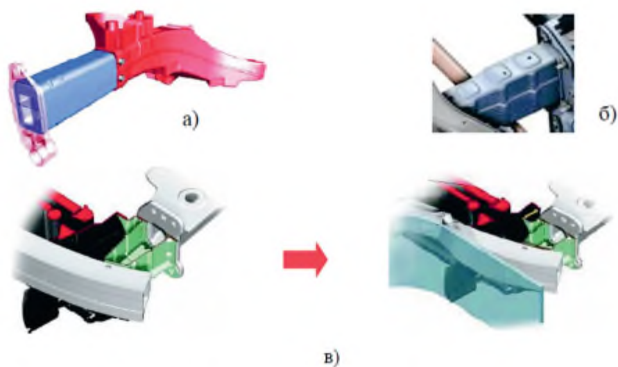
Крашбоксы с заломами Audi A2 (а), с готовыми складками Mercedes ML (б) и Audi A3 (в)
