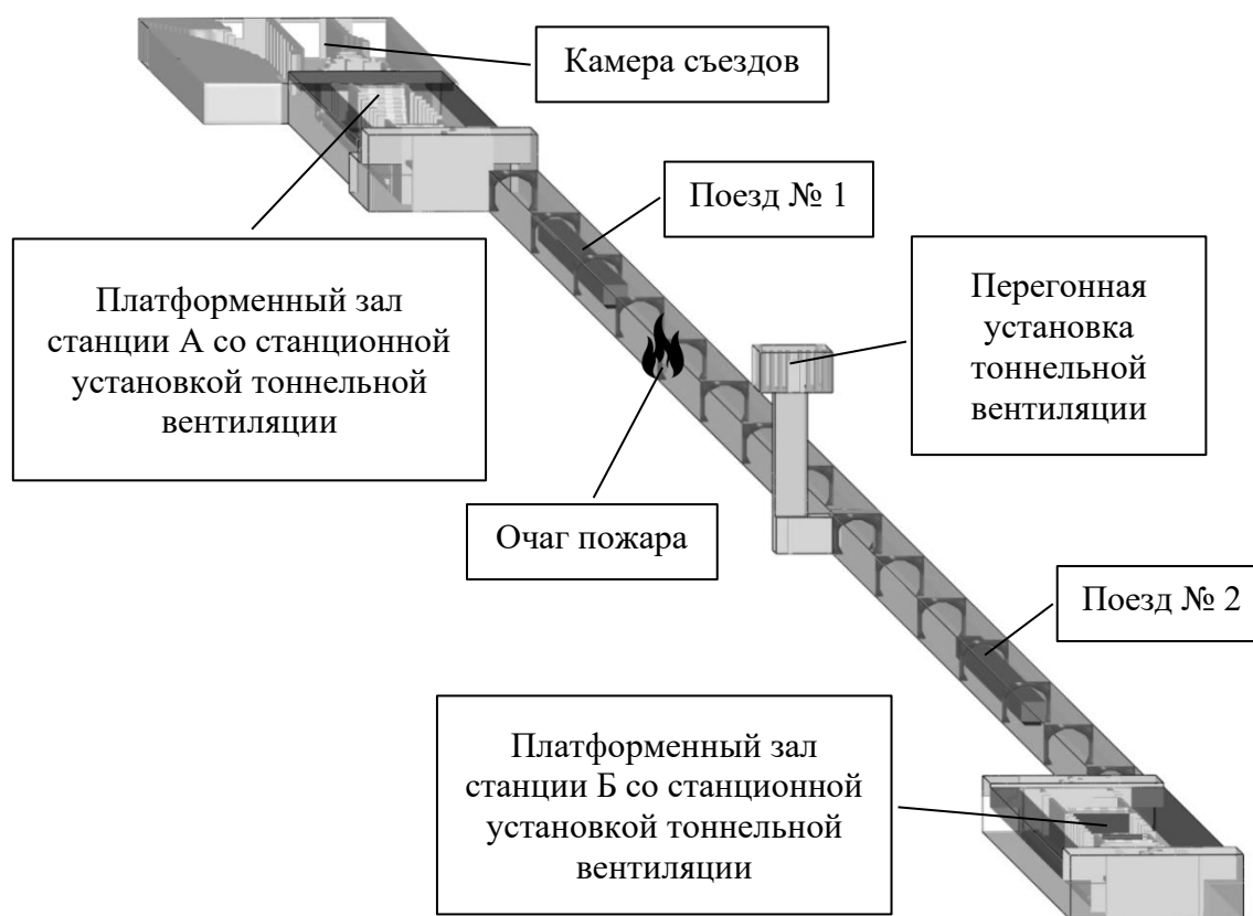
Рисунок 5.7 – Пример построения комплексной модели
