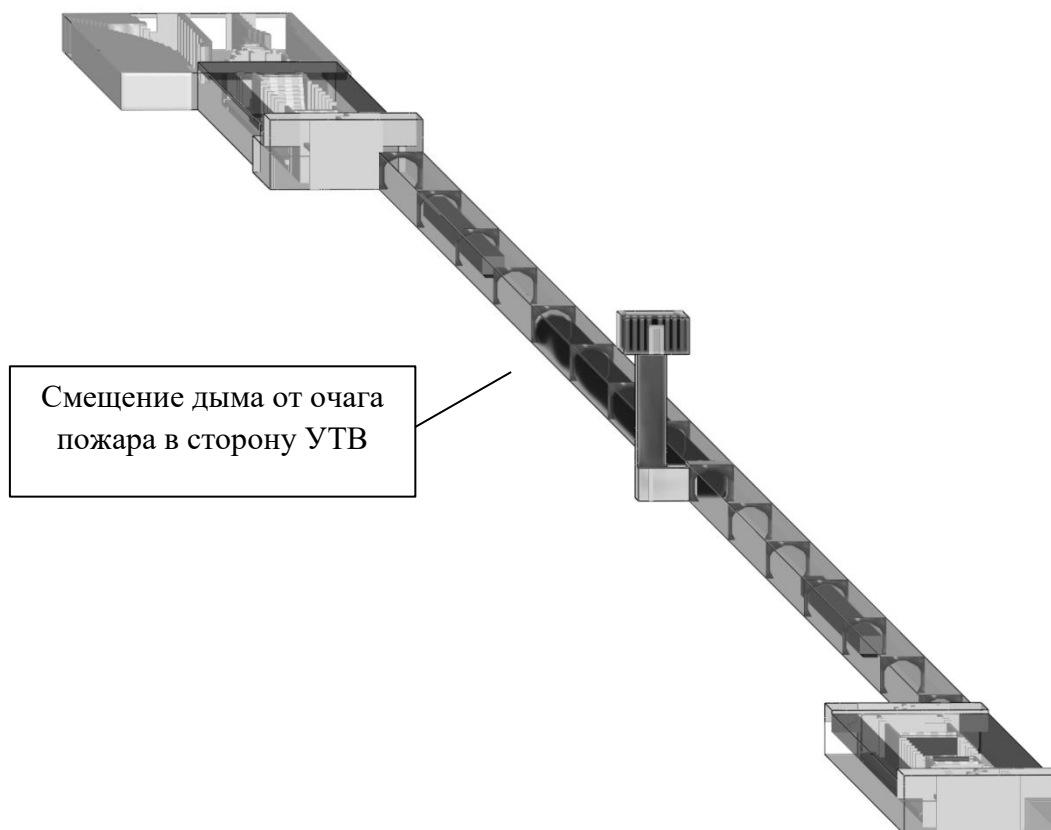
Рисунок 5.8 – Смещение дыма по примеру комплексной модели
