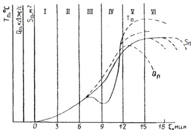
Рис. 7. Изменение основных параметров пожара во времени
