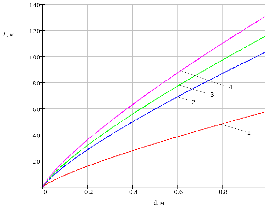
Рисунок 4.23 – Зависимость длины факела метана от диаметра трубопровода:
