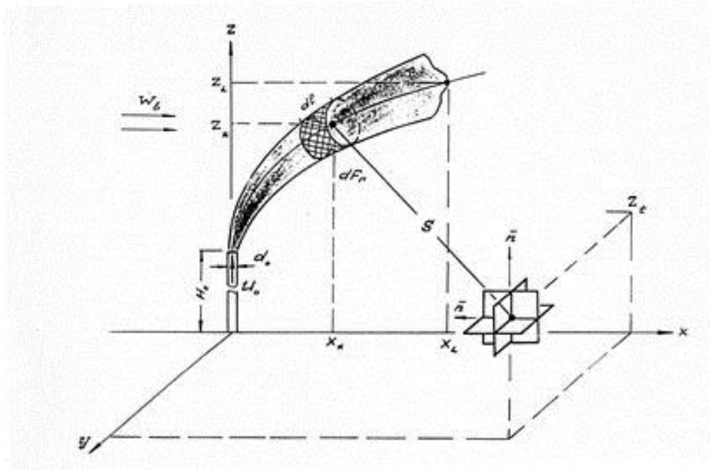
Рисунок 2.4 – К расчету модели линейно-поверхностного источника теплового излучения от струйного пламени
