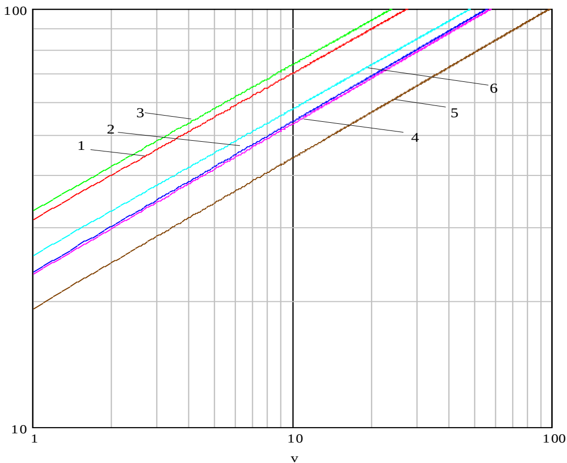
Рисунок 4.19 – Безопасное расстояние для рассматриваемых объектов при пожаре пролива СПГ, СУГ и водорода в зависимости от количества пролитого:
