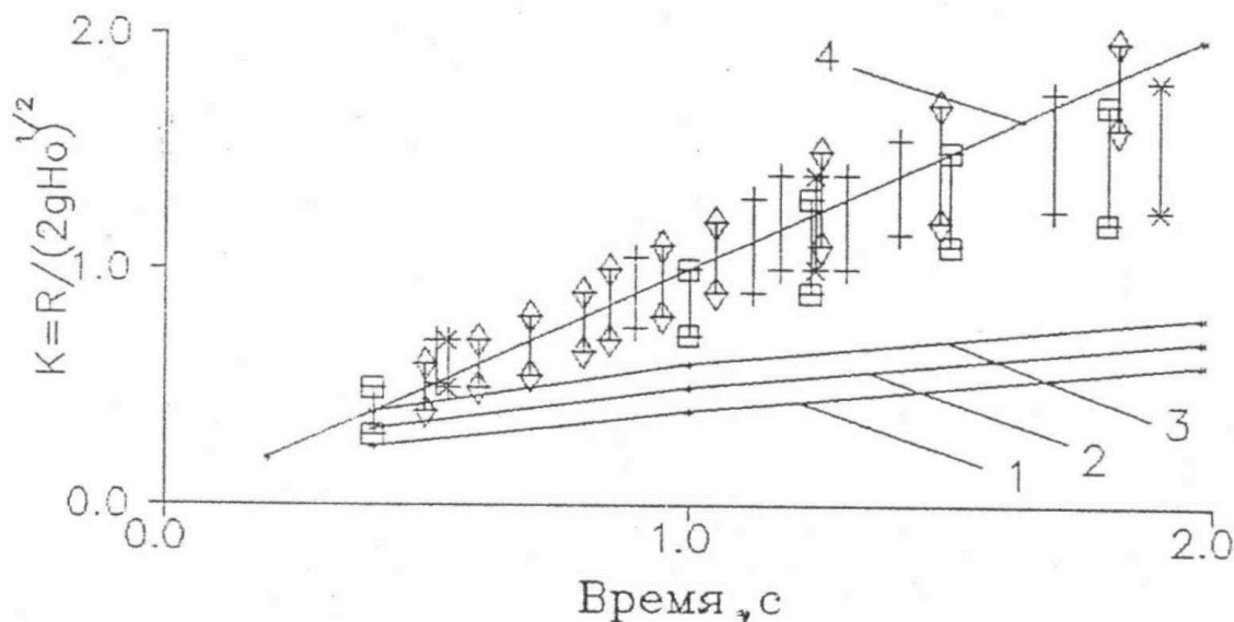
Рисунок 2.8 – Зависимость комплекса K = R / (2 \cdot g \cdot H_0)^{1/2} от времени при растекании водорода;
