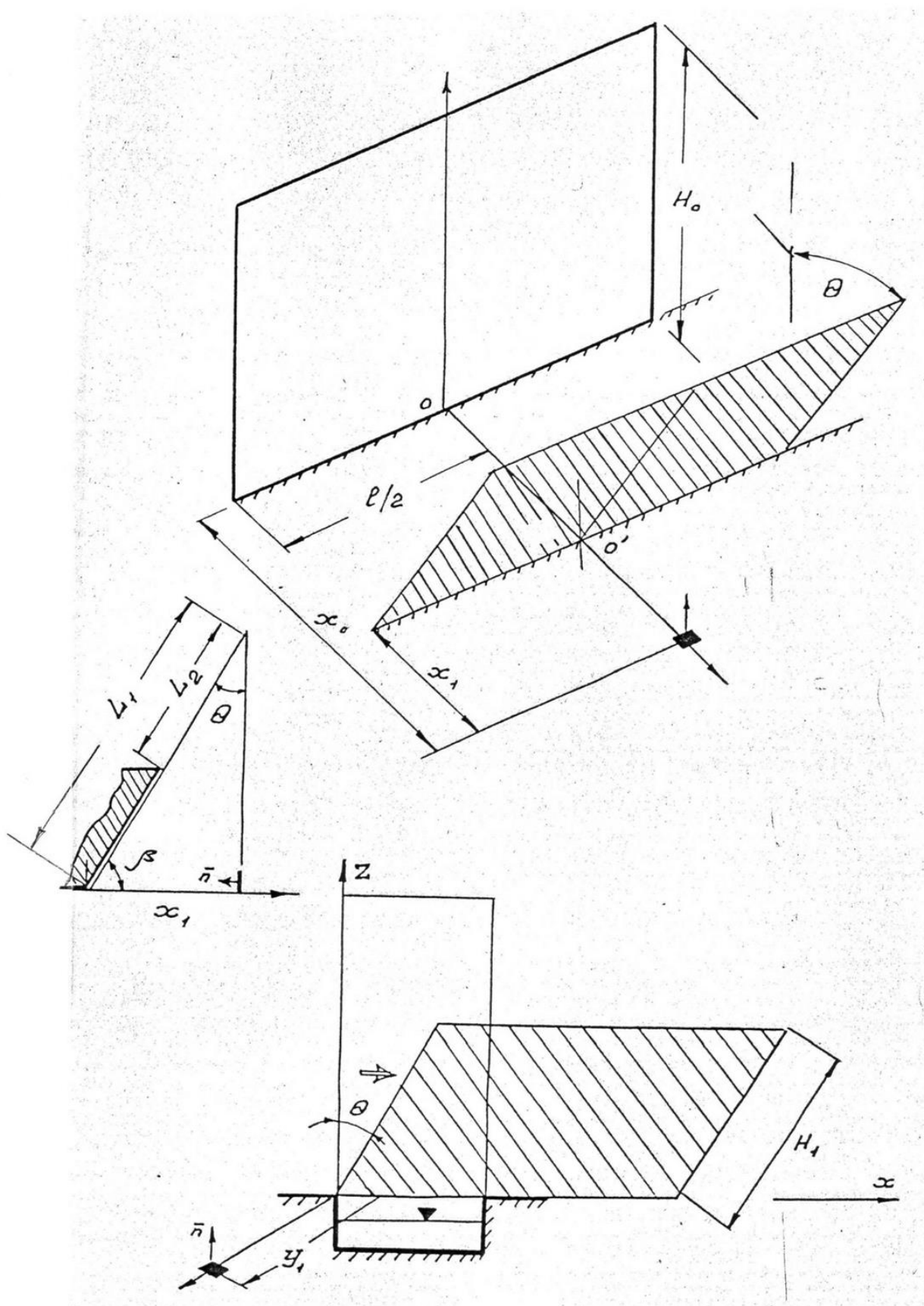
Рисунок 2.16 – К расчету угловых коэффициентов облучения
