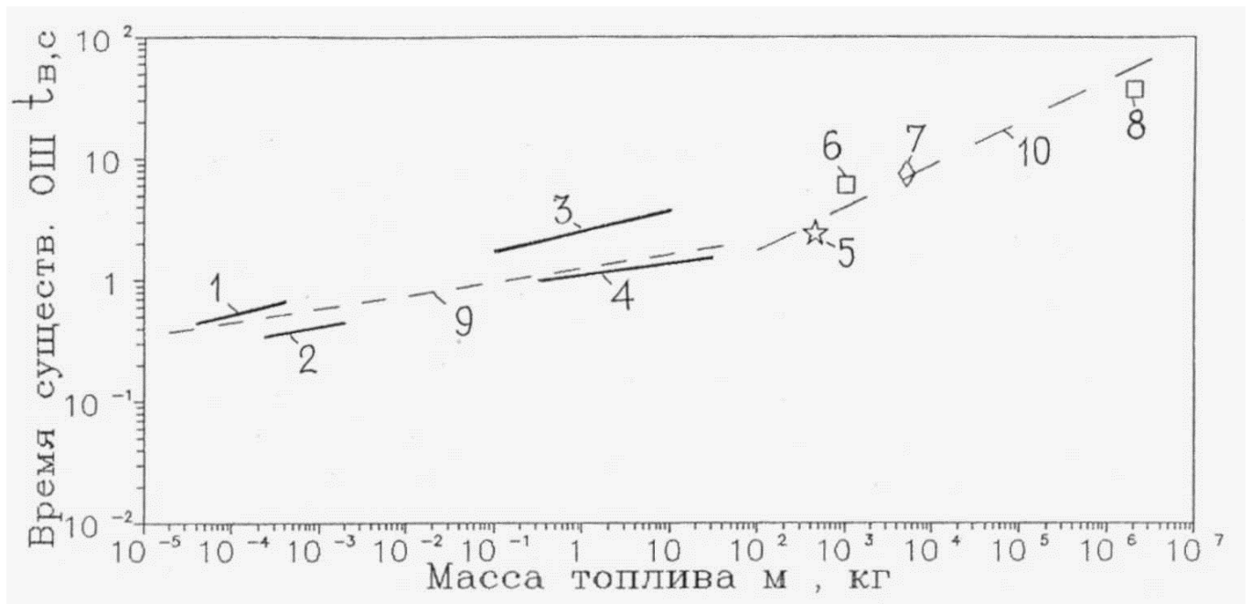
Рисунок 2.28 – Зависимость времени существования ОШ от массы топлива: 1 – пропан [14]; 2 – бутан [15]; 3 – метан [9]; 4 – пропилен, пентан, октан [8]; 5 – пропилен [6]; 6 – жидкий водород [16]; 7 – керосин + жидкий кислород [12]; 8 – взрыв ракеты «Сатурн-V» [11]; 9 – прямая t_b = 1,1m^{0,1} ; 10 – прямая t_b = 0,45m^{1/3}
