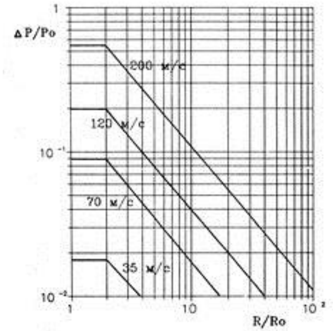
Рисунок 2.23 — Зависимость относительно избыточного давления в воздушной ударной волне сжатия от относительного расстояния при дефлаграции
