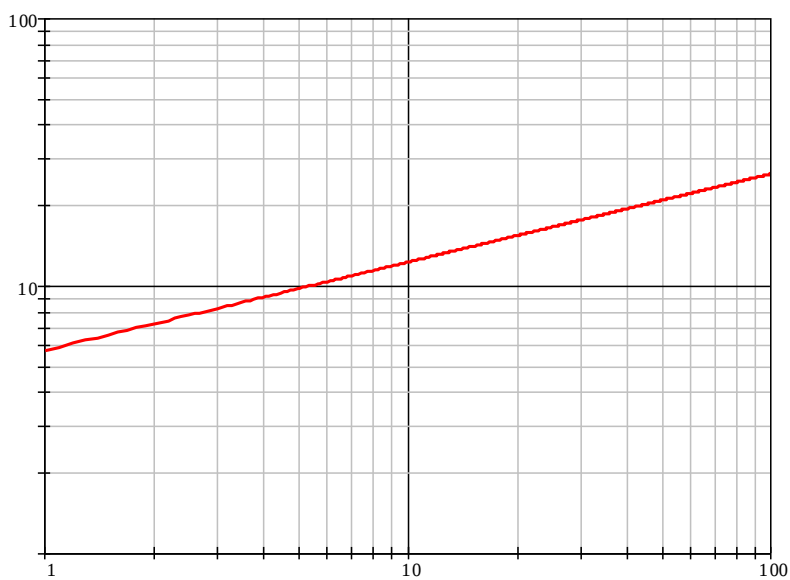
Рисунки 4.3 и 4.4 – Зависимость радиуса воздействия высокотемпературных продуктов сгорания паровоздушного облака ацетона при «пожаре-вспышке» от объема паров, вышедшего в атмосферу в результате аварии
