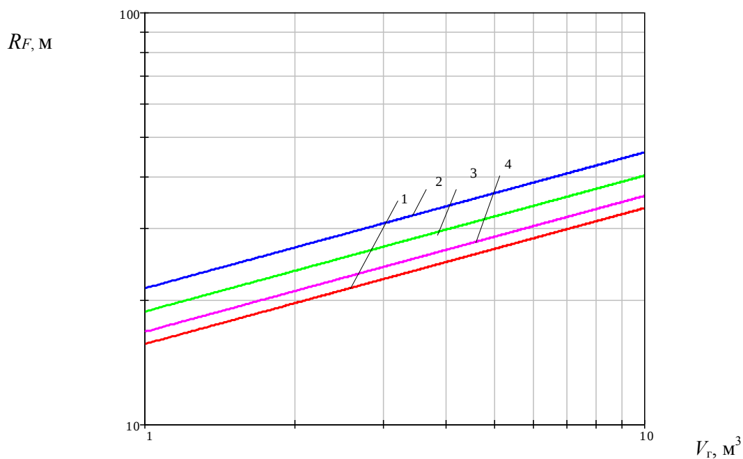
Рисунки 4.1 и 4.2 – Зависимость радиуса воздействия высокотемпературных продуктов сгорания газозвоздушного облака при «пожаре-вспышке» от объема газа, вышедшего в открытое пространство в результате аварии, V_g, \text{ м}^3 ; 1 – для облака смеси метана с воздухом; 2 – для облака смеси пропана с воздухом; 3 – для облака смеси этана с воздухом; 4 – для облака смеси водорода с воздухом;
