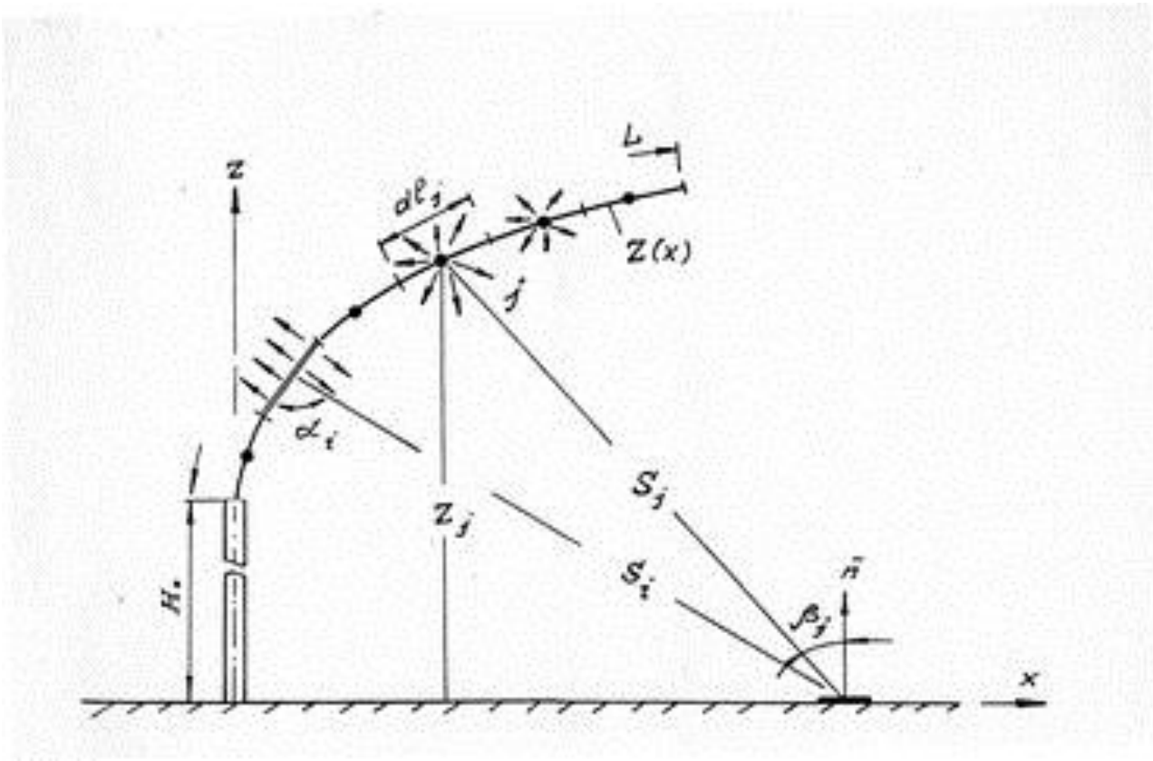
Рисунок 2.2 – К расчету модели многоточечного (линейного) источника теплового излучения от струйного пламени
