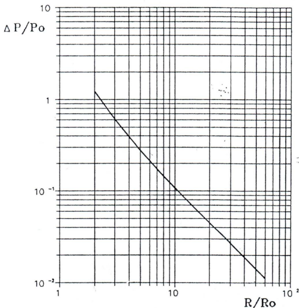
Рисунок 2.24 — Зависимости относительного избыточного давления в воздушной ударной волне сжатия от относительного расстояния при детонации
