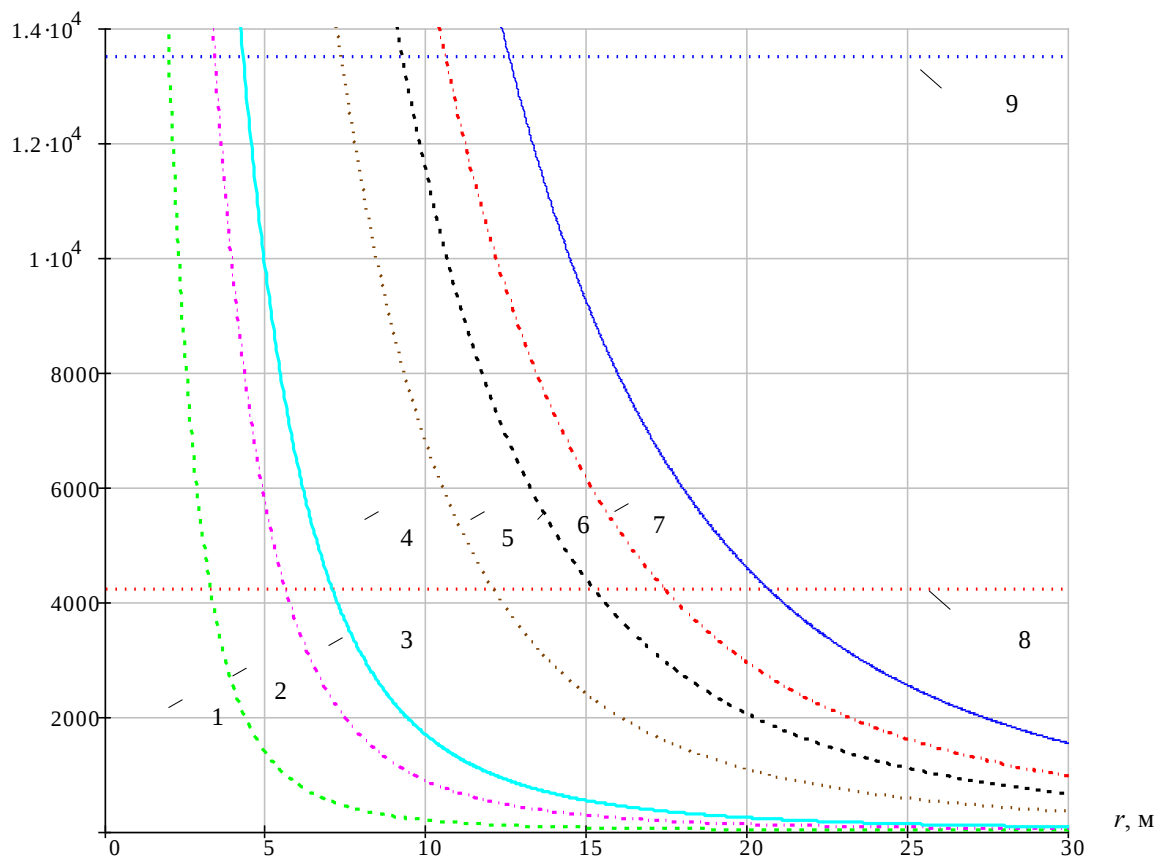
Рисунок 4.20 – Зависимость интенсивности теплового излучения огненного шара на расстоянии r от точки на поверхности земли непосредственно под центром огненного шара: 1 – масса горючего m=0,1 кг; 2 – m = 0,5 кг; 3 – m = 1 кг; 4 – m = 5 кг; 5 – m = 10 кг; 6 – m = 15 кг; 7 – m = 25 кг; 8 – критическое пороговое значение интенсивности теплового излучения для человека, равное 4,2 \text{ кВт/м}^2 ; 9 – критическое пороговое значение интенсивности теплового излучения для зданий, сооружений и наружных установок, равное 13,5 \text{ кВт/м}^2
