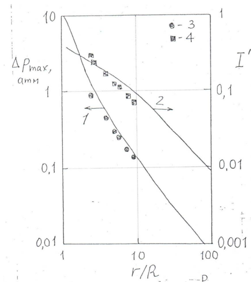
Рисунок 2.22 – Сравнение расчетов по модели Бринкли – Кирквуда: 1, 2 – расчетные кривые для давления и импульса; 3, 4 – экспериментальные данные [14].
