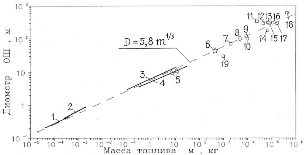
Рисунок 2.27 – Зависимость диаметра огненного шара от массы топлива:
