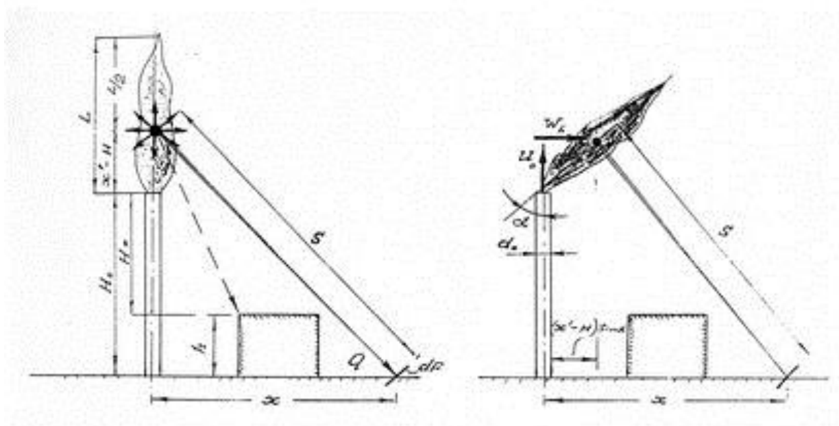
Рисунок 2.1 – К расчету воздействия факела на окружающую среду – модель Т. Бжустовски
