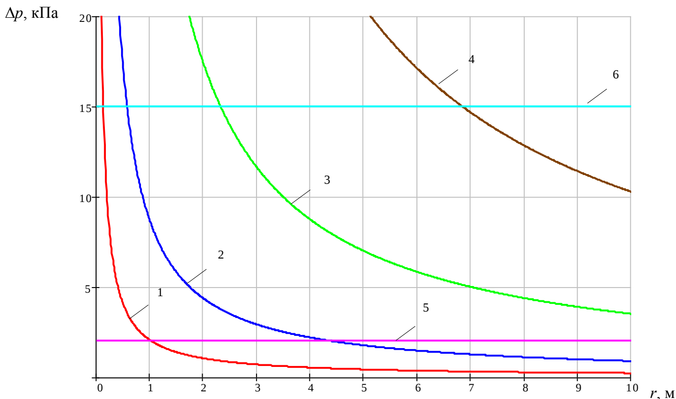
Рисунок 4.10 – Зависимость избыточного давления в УВ от расстояния от центра взрыва при различных загроможденностях окружающего пространства:
