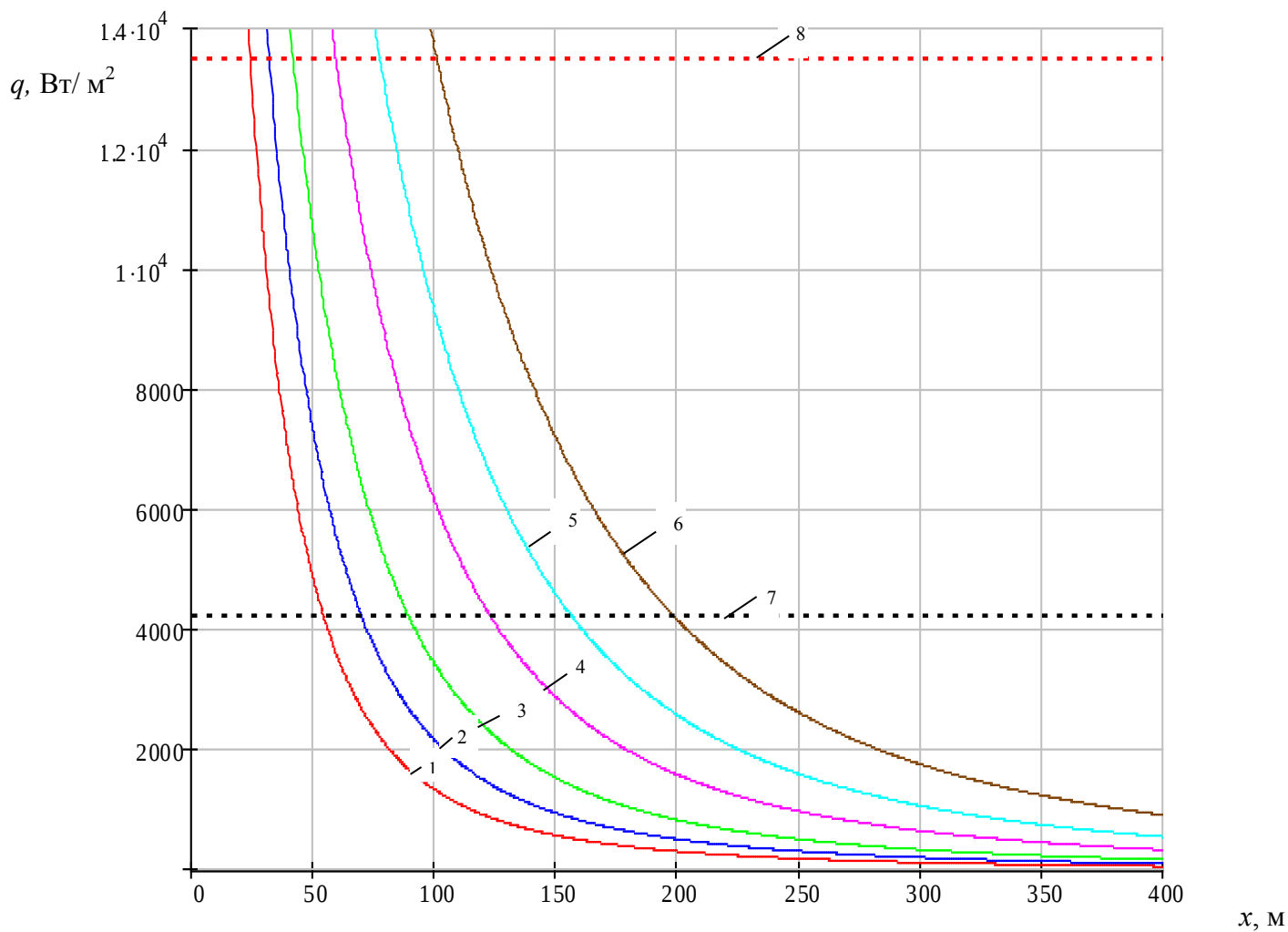
Рисунок 4.16 – Интенсивность теплового излучения на расстоянии x , м от пожара пролива СПГ: 1 – пролив 5 \text{ м}^3 СПГ; 2 – пролив 10 \text{ м}^3 СПГ; 3 – пролив 20 \text{ м}^3 СПГ; 4 – пролив 50 \text{ м}^3 СПГ; 5 – пролив 100 \text{ м}^3 СПГ; 6 – пролив 200 \text{ м}^3 СПГ; 7 – пороговое значение интенсивности теплового излучения для человека, равное 4,2 \text{ кВт/м}^2 ; 8 – пороговое значение интенсивности теплового излучения для зданий, сооружений, равное 13,5 \text{ кВт/м}^2
