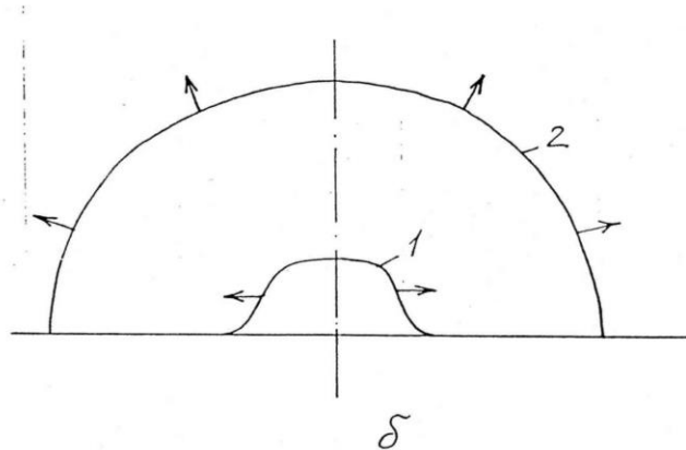
Рисунок 2.20 – Схема Пикле для расчета дефлаграционного сгорания дискообразного облака. Расчетная модель: 1 – поршень, 2 – фронт взрывной волны
