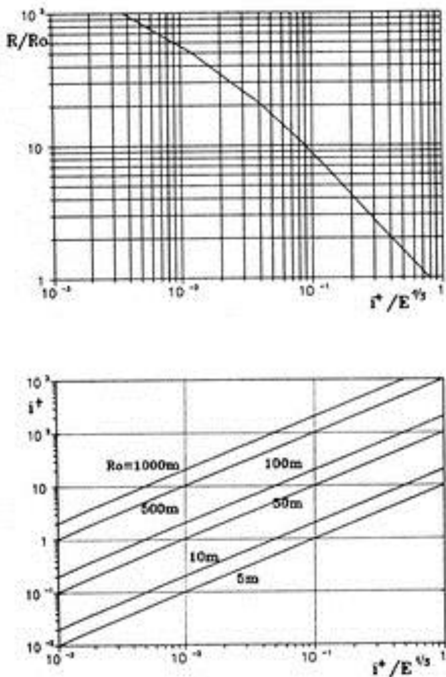
Рисунок 2.25 Зависимости приведенного импульса от относительного расстояния и импульса для различных начальных размеров пожароопасных облаков при детонации
