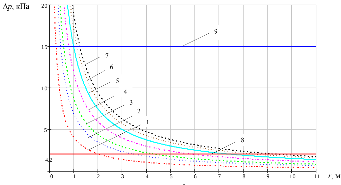
Рисунок 4.9 – Зависимость избыточного давления в ударной волне от расстояния до объекта, при дефлаграционном сгорании облака метановоздушной смеси в среднезагроможденном пространстве при различных значениях V :
